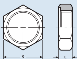
Hex. Nut / 6-Kant Mutter / Ecrou hex. / Zeskant
