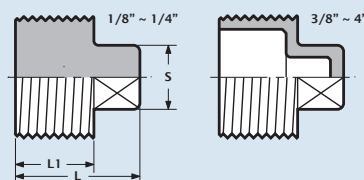
Sqare plug / 4-Kant Stopfen / Bouchon à tête carrée / Vierkant stop
