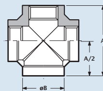
Cross / Kreuzstück / Croix / Kruisstuk
