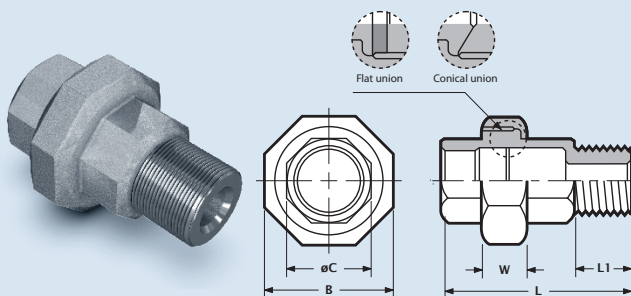
Union M-F conicle-flatsealing / Verschraubung I-A konisch-flachdichtend / Raccord union M-F conique-joint teflon / Koppeling bi-bu conisch-vlakdichtend /
