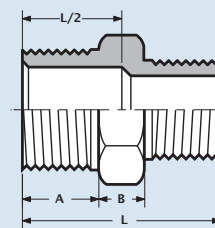
Red. hex nipple / 6-Kant Reduziertnippel / Réduction hexagonale / Verloop nippel
