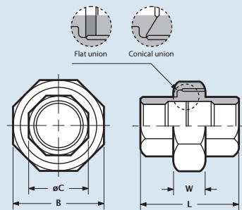
Union conicle-flatsealing / Verschraubung konisch-flachdichtend / Raccord union joint plat teflon / Koppeling conisch-vlakdichtend
