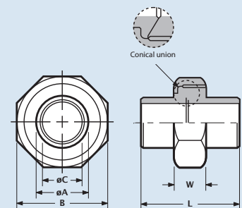
Union for welding conicle / Verschraubung Anschweißende / Raccord a souder conique / Laskoppeling conisch
